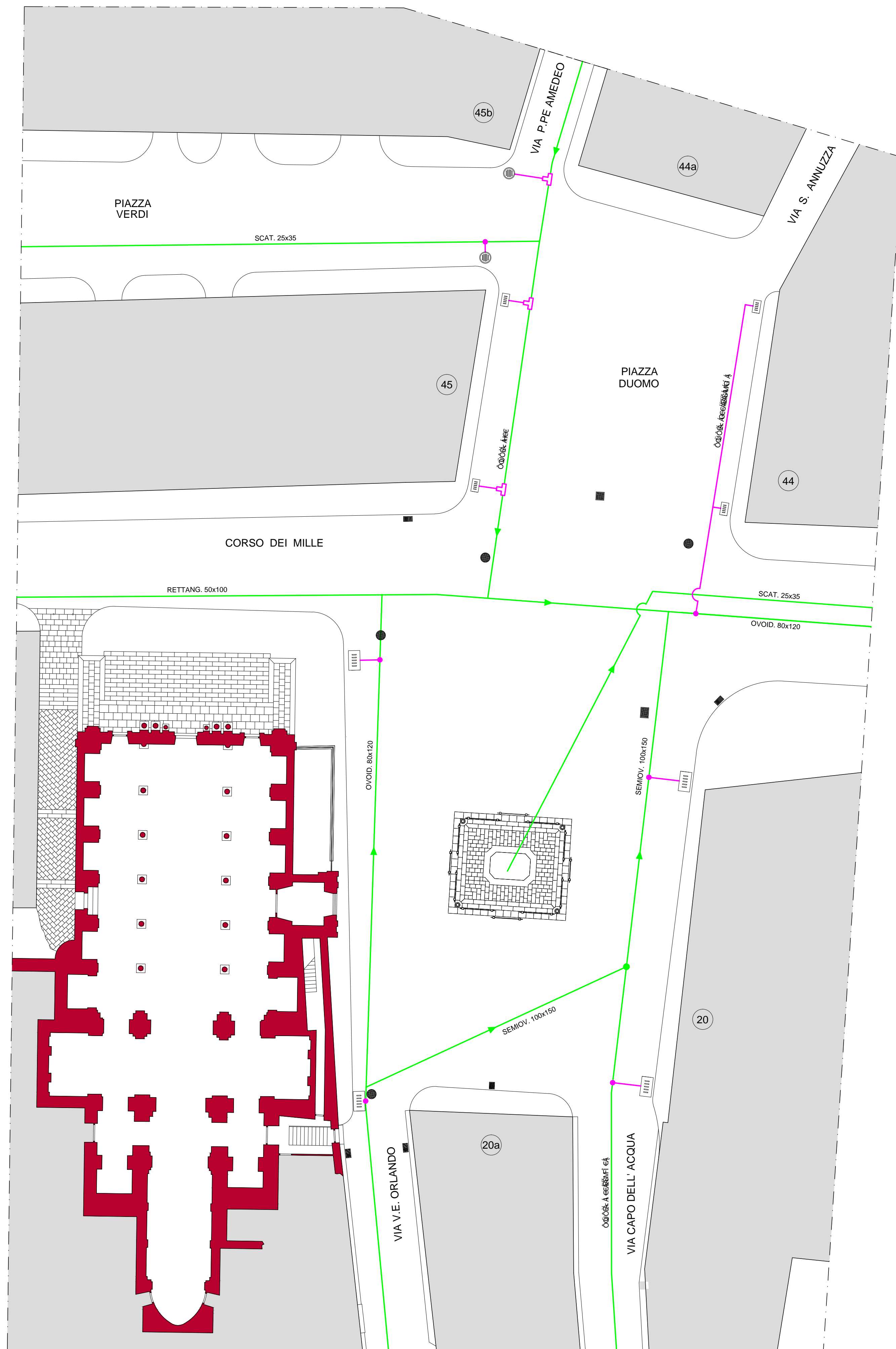
PLANIMETRIA GENERALE RETE FOGNANTE STATO DI PROGETTO
